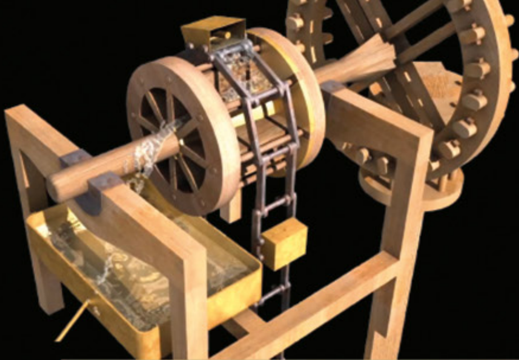
Recreación en 3D del Artificio de Toledo a partir de la versión de Ladislao Reti (Fundación Juanelo Turriano)
